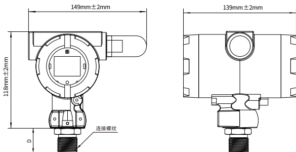
图 1 产品外形尺寸
