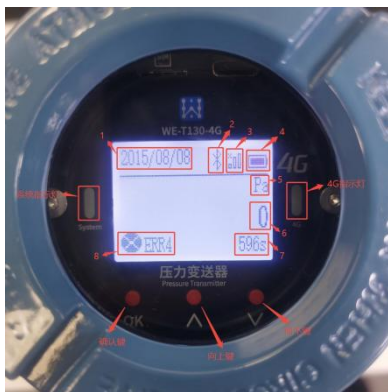
图3 面板示意图
