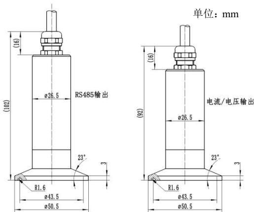
图2 常温直接引线式（卡箍连接）
