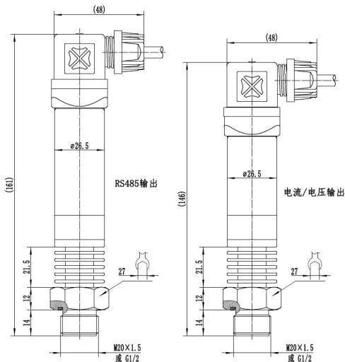
图 11 高温赫斯曼式（螺纹连接，5 片散热片）
