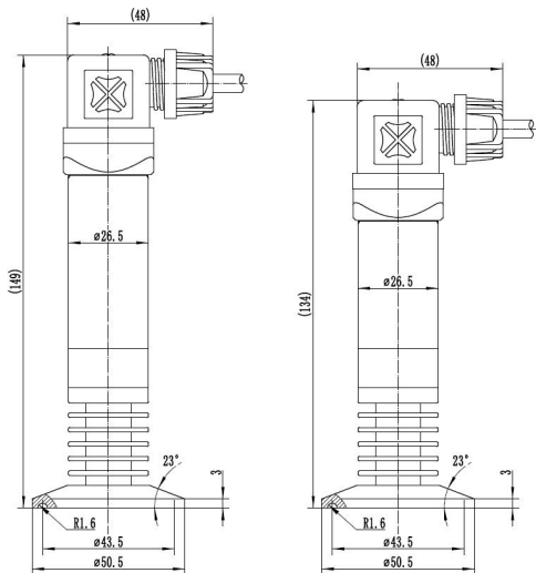
图 12 高温赫斯曼式 (卡箍连接, 5 片散热片)
