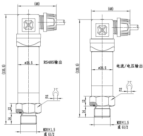
图 5 常温赫斯曼式（螺纹连接）
