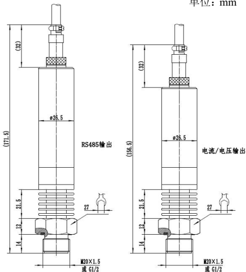
图 9 高温航插式（螺纹连接，5 片散热片）
