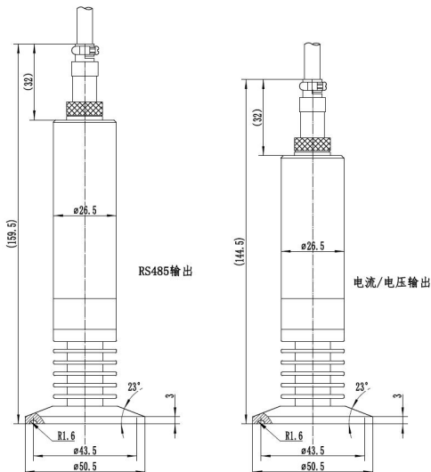
图 10 高温航插式 (卡箍连接, 5 片散热片)
