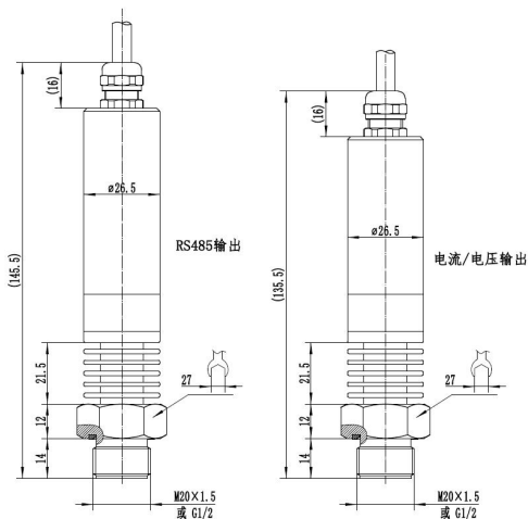
图 7 高温直接引线式（螺纹连接，5 片散热片）
