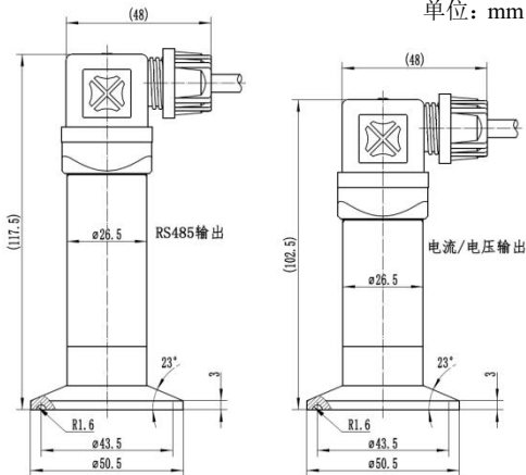
图 6 常温赫斯曼式 (卡箍连接)
