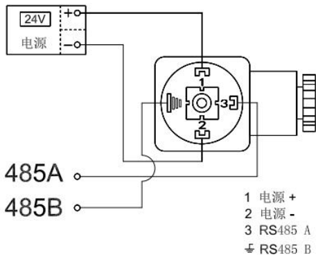
图 17 RS485 输出接线示意
