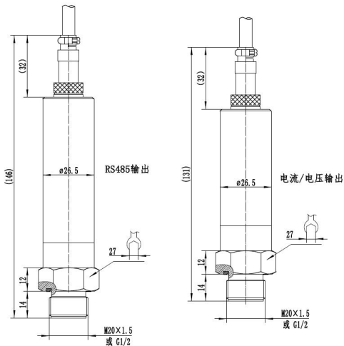
图 3 常温航插式（螺纹连接）
