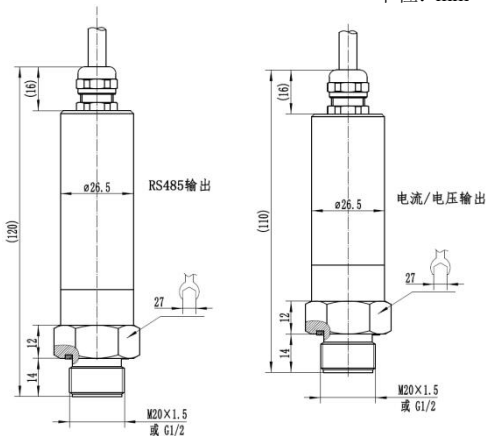
图 1 常温直接引线式（螺纹连接）
