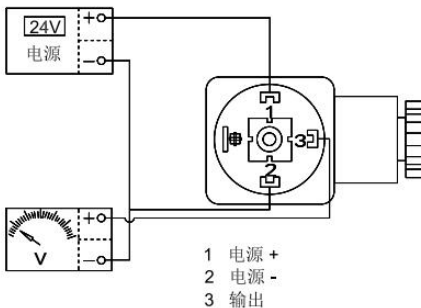
图 16 电压输出接线示意
