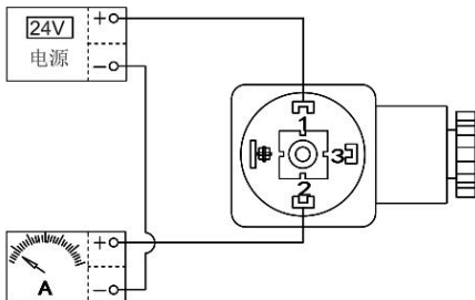
图 15 二线制电流输出接线示意
