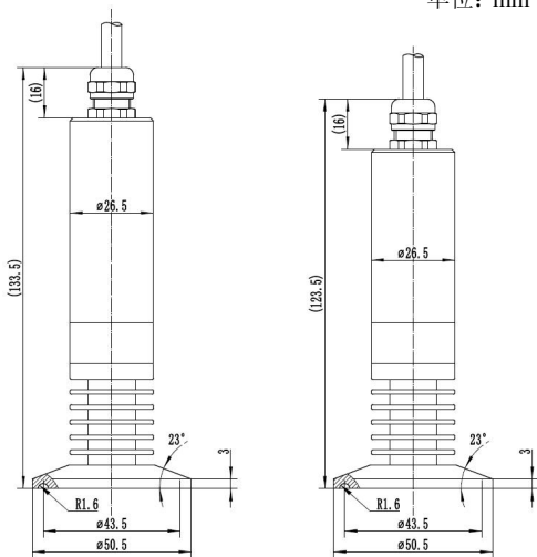
图 8 高温直接引线式（卡箍连接，5 片散热片）
