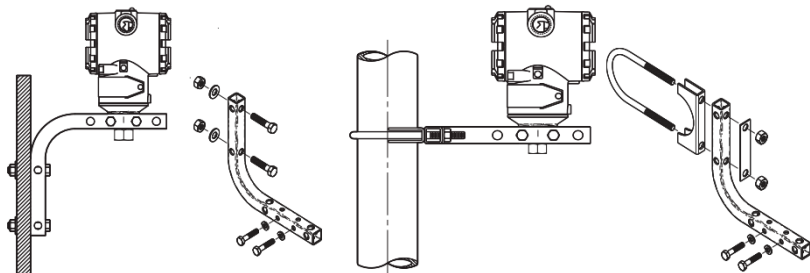
图 2-2 单晶硅压力变送器安装
