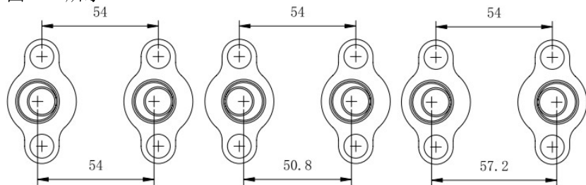
图 2-5 差压变送器连接孔距图
