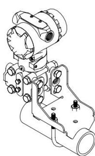
B1 管装弯支架
