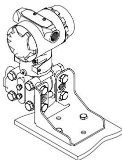
B2 盘装弯支架
