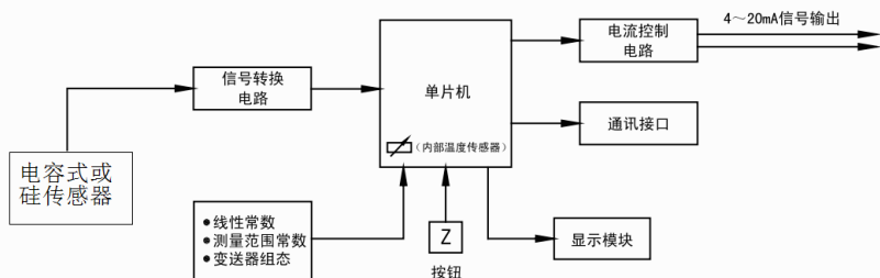
图 1-1 变送器原理框图
