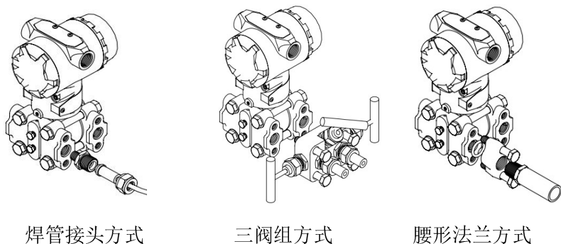
图 2-4 单晶硅差压变送器引压图
